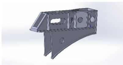
Н125 кронштейн шлюпбалки зад.
